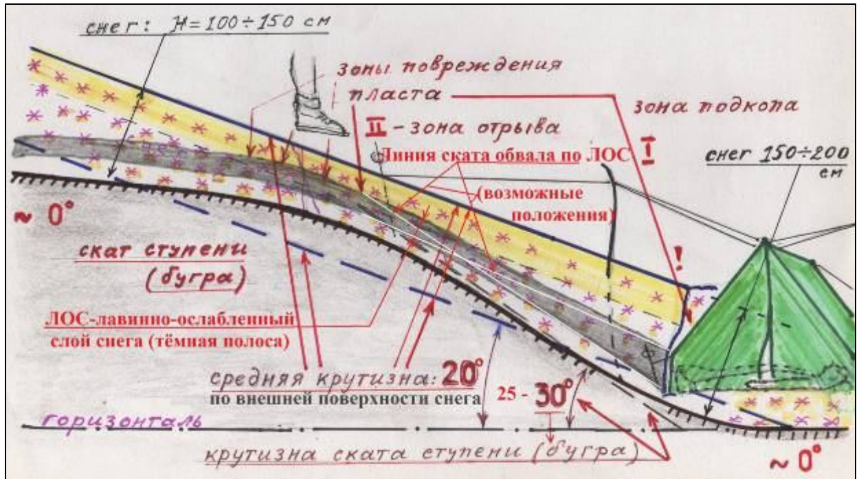
Рисунок 2. Возможное положение линий «ската» показано белыми линиями на тёмной полосе, обозначающей слой разрыхления под «снежной доской»
